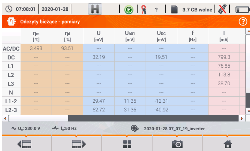
Rys. 47. Odczyty bieżące w widoku tabelarycznym w trybie pomiaru sprawności inwertera.
