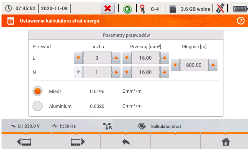
Rys. 50. Analiza strat energii – ekran konfiguracyjny 1
